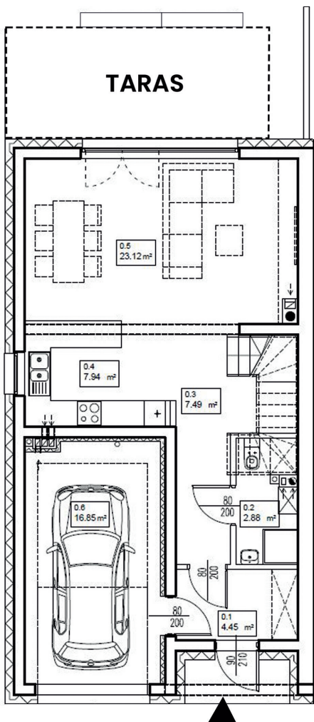
RZUT PARTERU
