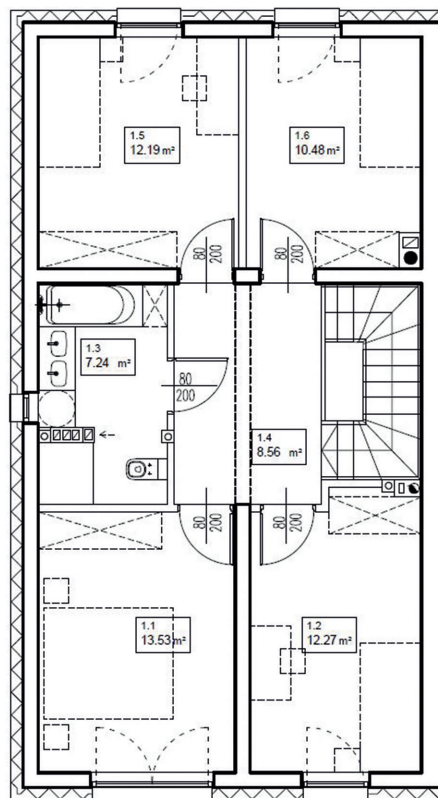
RZUT PIĘTRA
