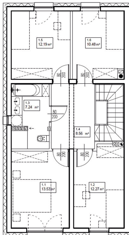
RZUT PIĘTRA
