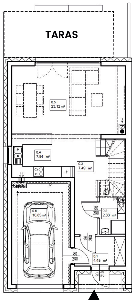
RZUT PARTERU
